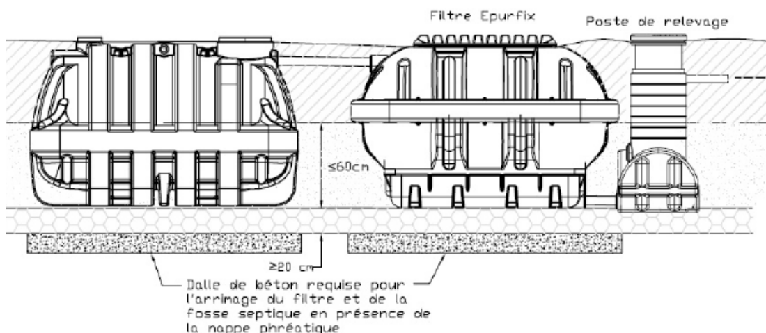
Figure 39 : conditions de nappe haute avec ancrage
