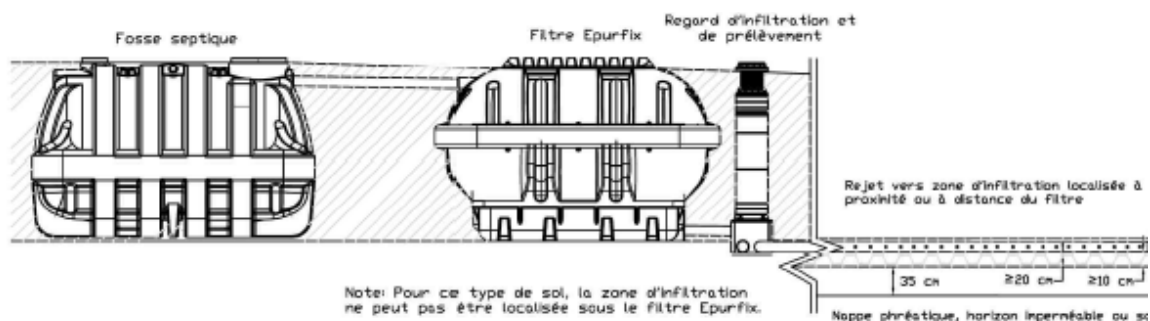
Figure 40 : conditions de sol limoneux avec infiltration distante
