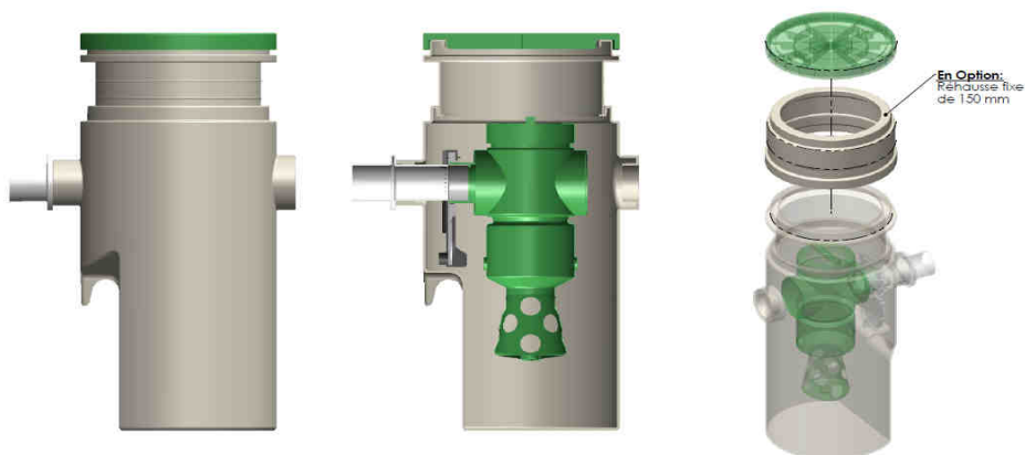
Figure 43 : Préfiltre dans sa boîte indépendante
