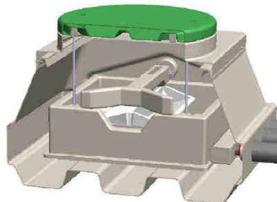
Figure 2 : Répartiteur 3 voies
