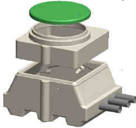
Figure 47 : Répartiteur avec réhausse et couvercle verrouillable
